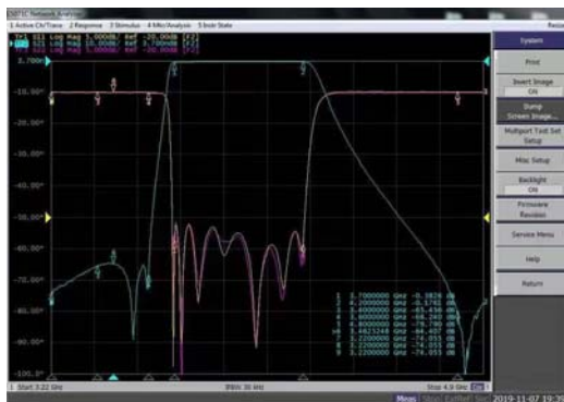
测试曲线图
